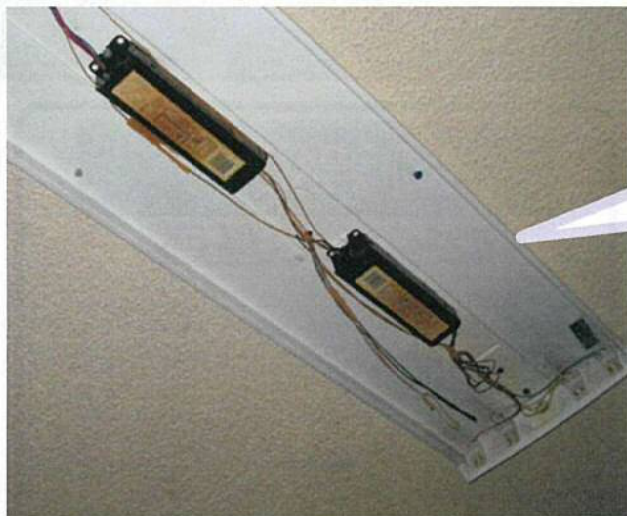
▼長期間の使用で内部が劣化した安定器
